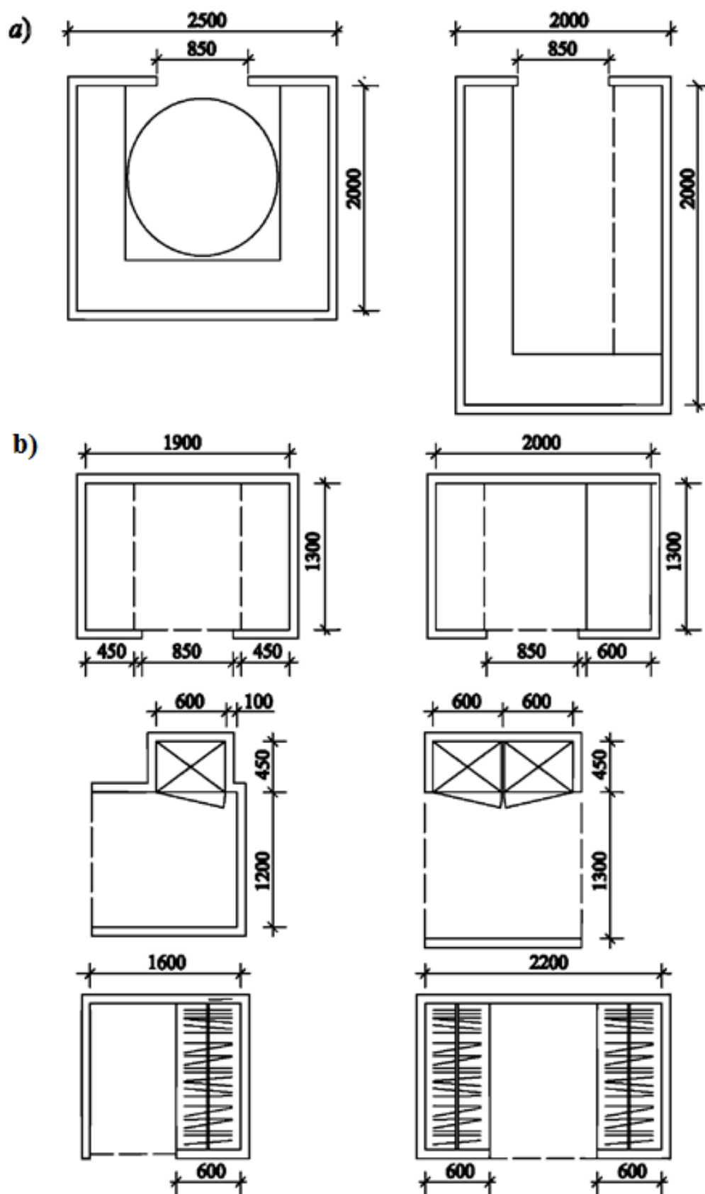
Figura A.8 – Depozite de produse alimentare (a) și depozite de uz casnic, dulapuri încorporate și vestiare (b)
