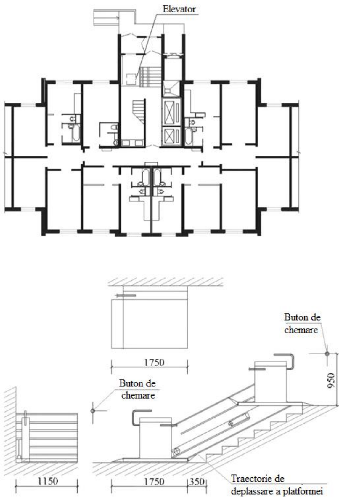
Figura A.3 - Decizii ale grupului vestibul - intrare cu instalarea elevatorului cu transport pe orizontală
