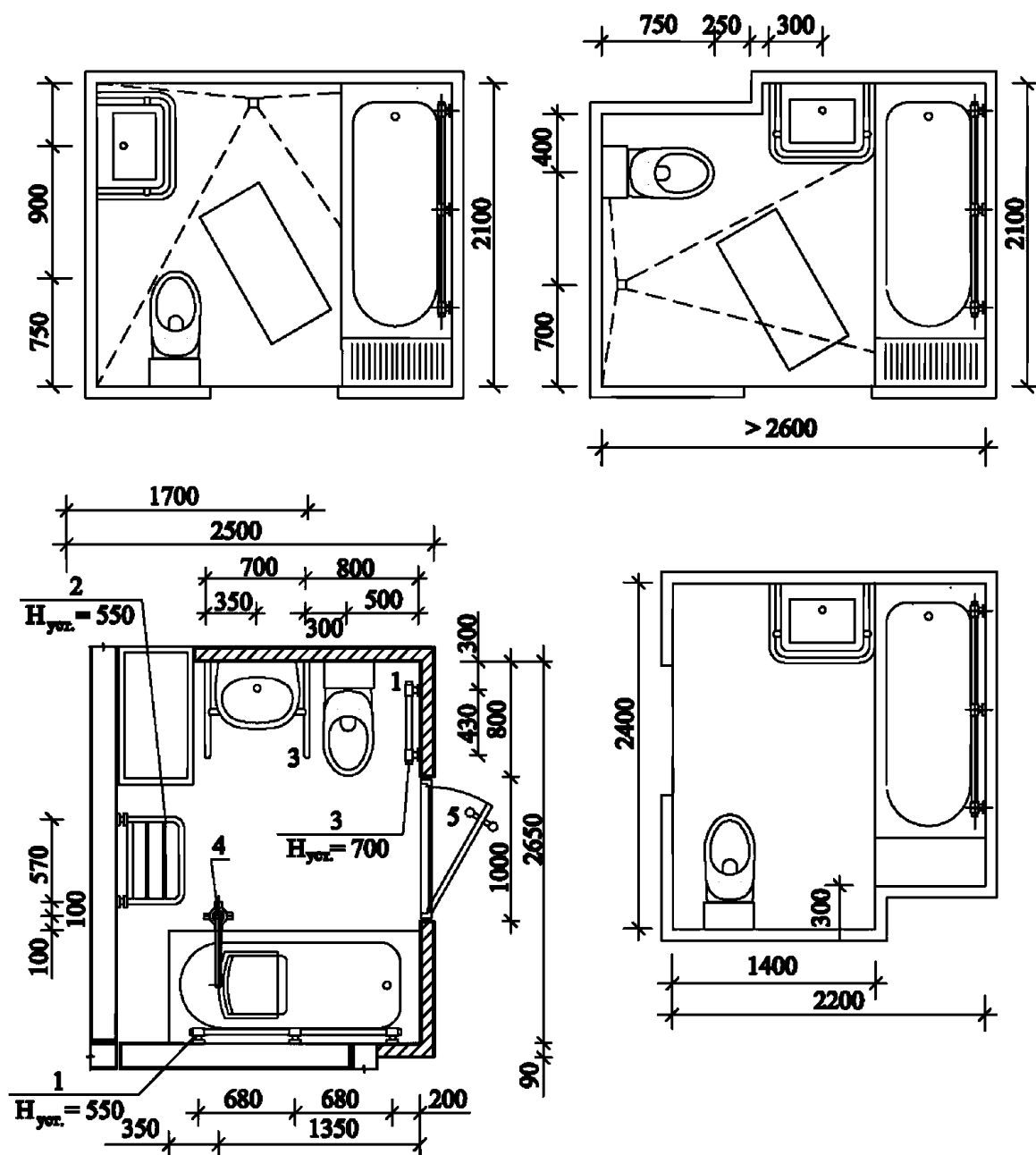
1 - поручень настенный; 2 - сиденье; 3 - поручень для умывальника; 4 - гидроподъемник; 5 - поручень ручка дверная Рисунок А.12 - Совмещенные санузлы, оборудованные ванной для инвалидов, пользующихся креслом-коляской
