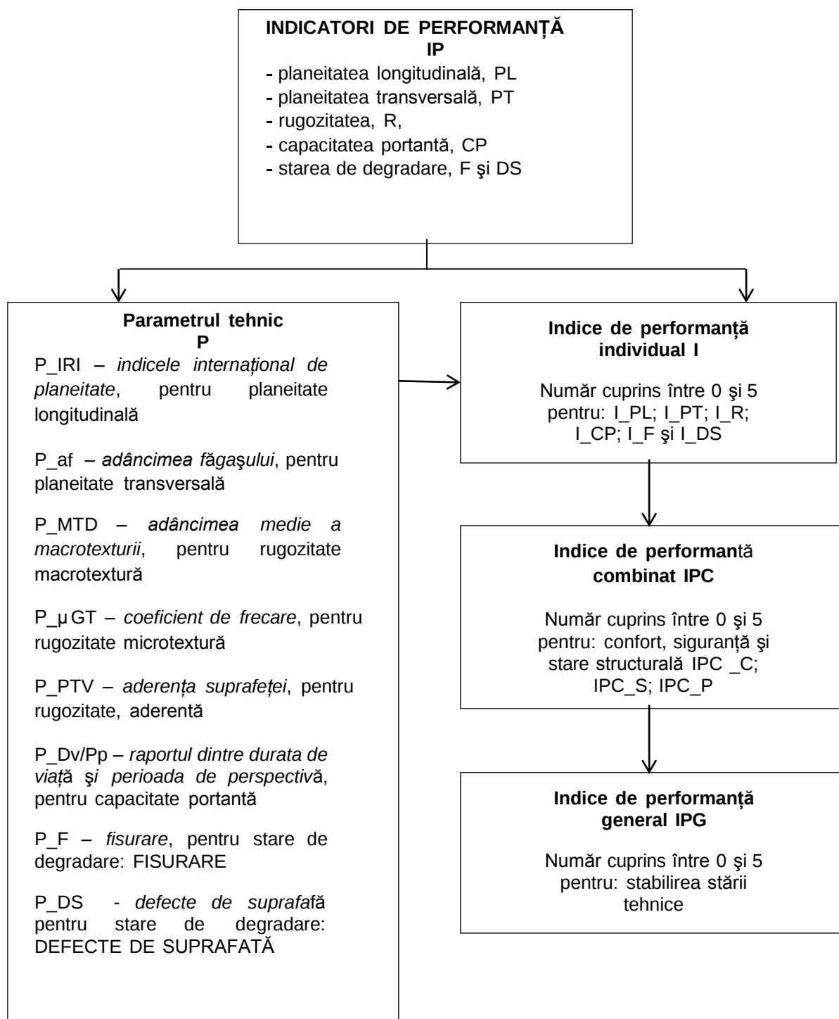
Figura 1 Scema sinoptică de satabilire a calificativului stării tehnice a drumurilor
