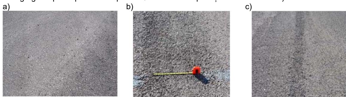
a) - nivel scăzut de severitate (S); b) - nivel mediu de severitate (M); c) - nivel ridicat de severitate (R)
