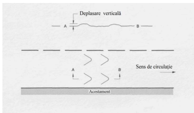
Figura 8 - Modul de măsurare a vălurilor
