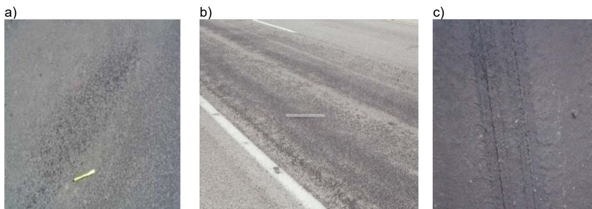
a) – nivel de severitate scăzut; b) – nivel de severitate mediu; c) – nivel de severitate ridicat
