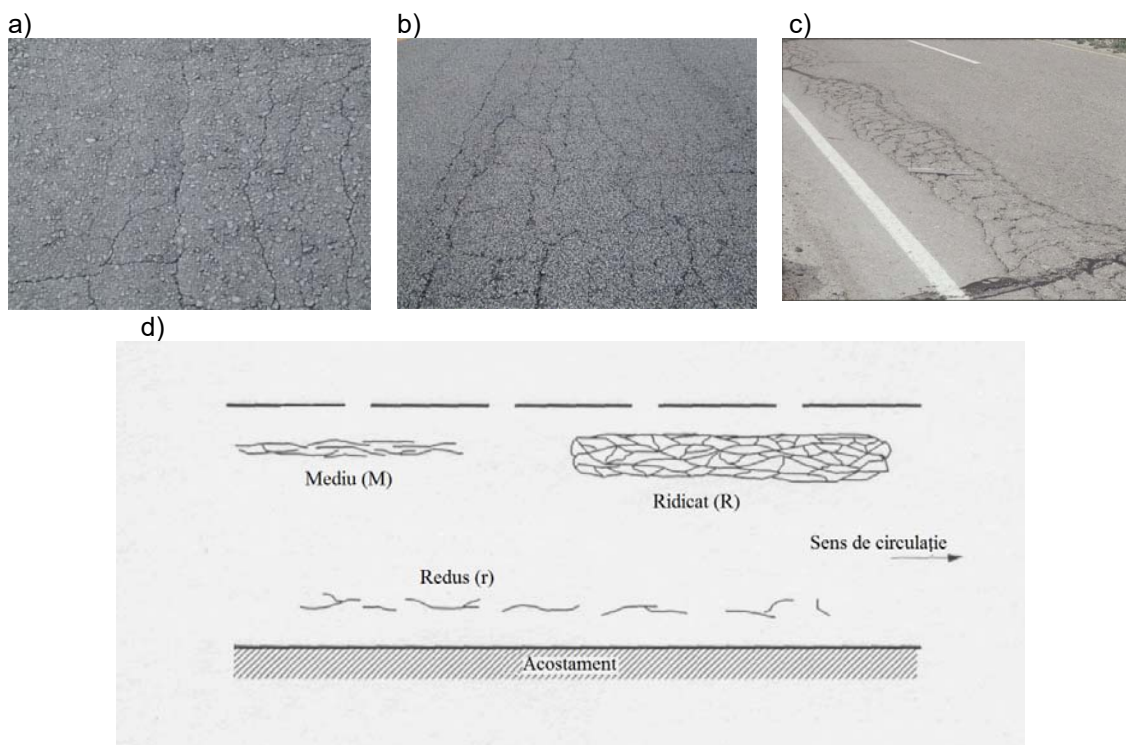
a) - nivel scăzut de severitate (S); b) - nivel mediu de severitate (M); c) - nivel ridicat de severitate (R); d – reprezentare schematică a nivelelor de severitate
