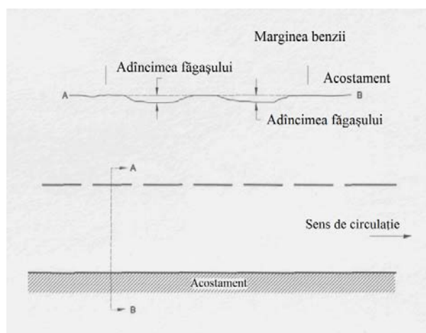
Figura 19 - Modul de măsurare a adâncimii fâgașelor
