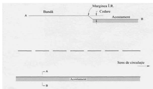
Figura 41 - Prezentarea schematică a cedării acostamentelor
