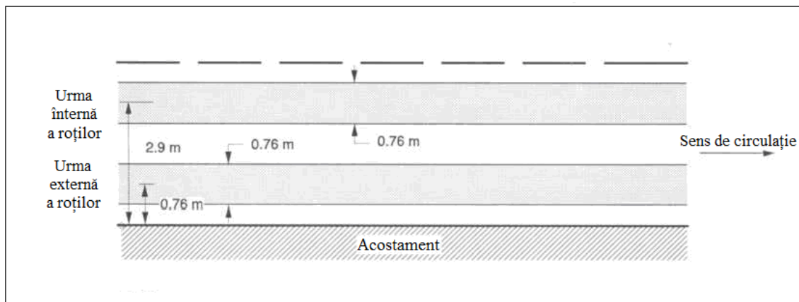
Figura 80 - Localizarea urmelor roţilor pe banda de rulare.
