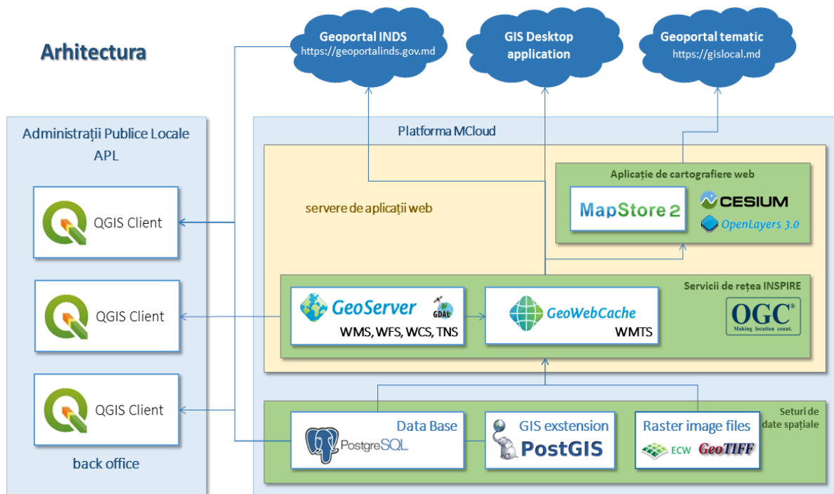
Fig. 1. Schema funcțională a SIGSNL și componentele acestuia
