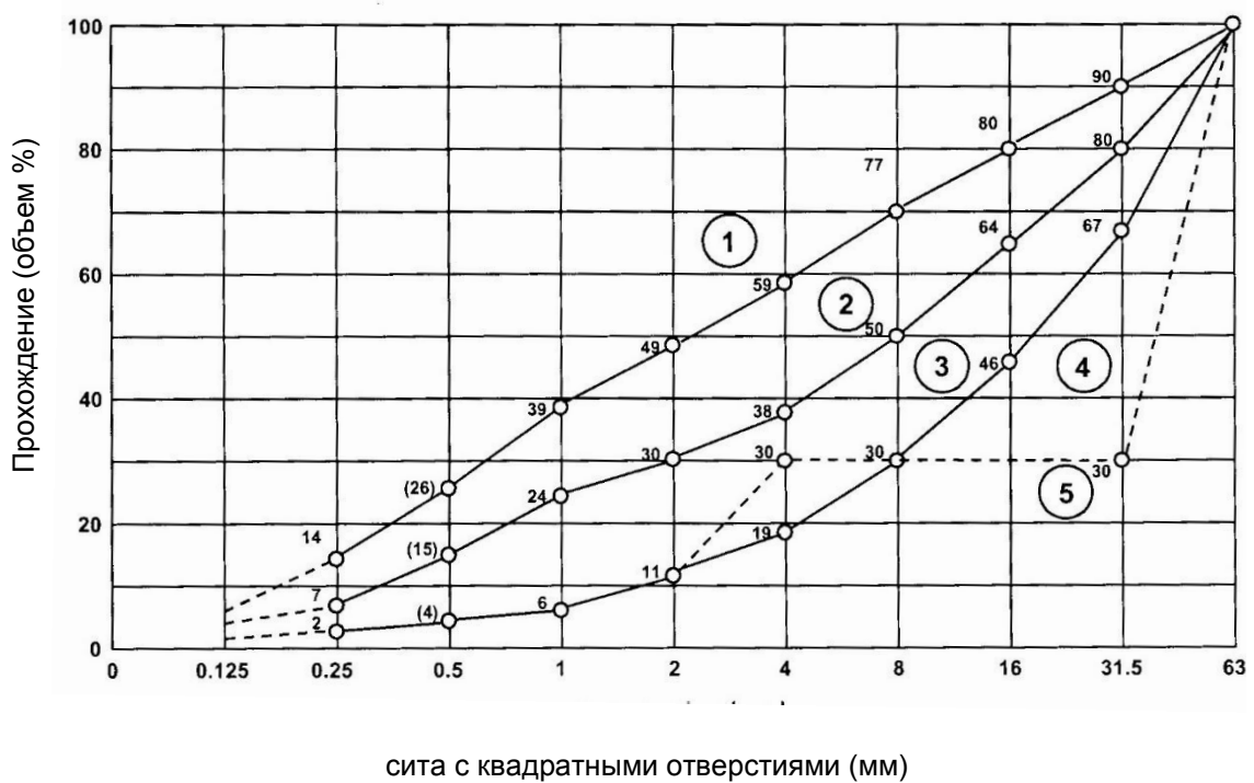
Рисунок J.4 - Гранулометрические области для максимального размера заполнителей 32 мм
