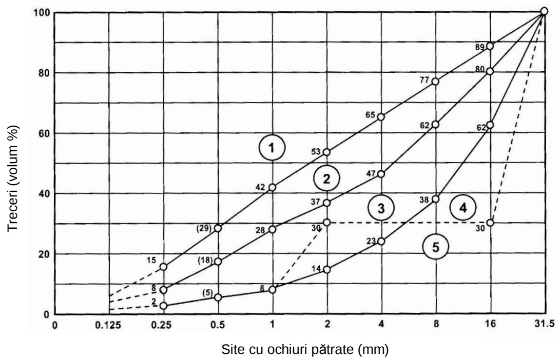
Figura J.3 - Zone de granulozitate pentru dimensiunea maximă a agregatelor de 22 mm
