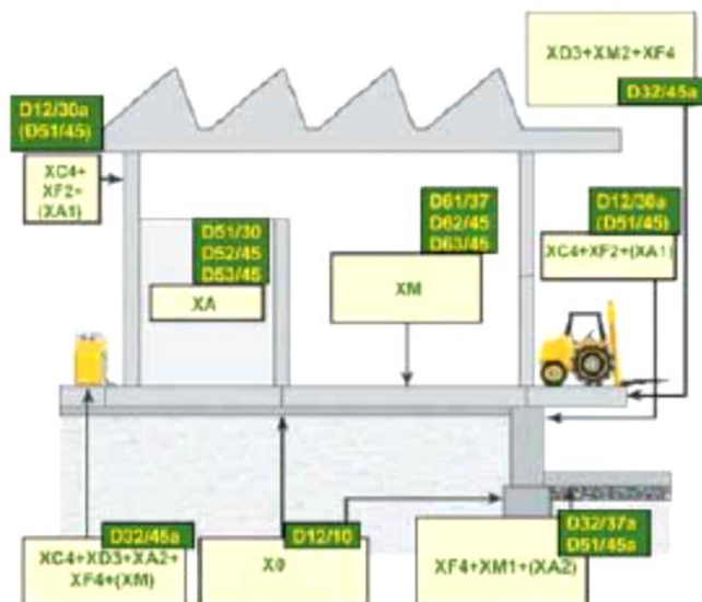
Рисунок V.3 - Примеры классов долговечности/комбинации классов сред эксплуатации (промышленные конструкции)
