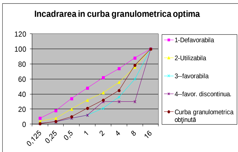
EXEMPLUL 2 - Zone de granulozitate pentru dimensiunea maximă a agregatelor de 32 mm determinată conform SM SR EN 933-1.
