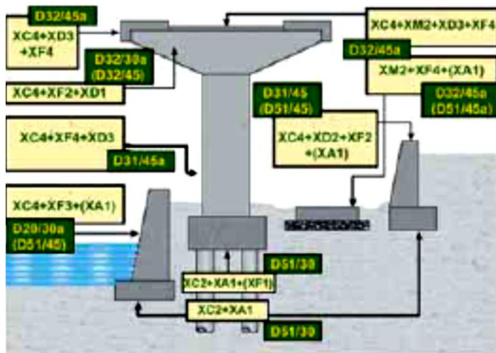
Рисунок V.2 - Примеры классов долговечности/комбинации классов сред эксплуатации (строительство дорог, мостов, гидротехнических сооружений)
