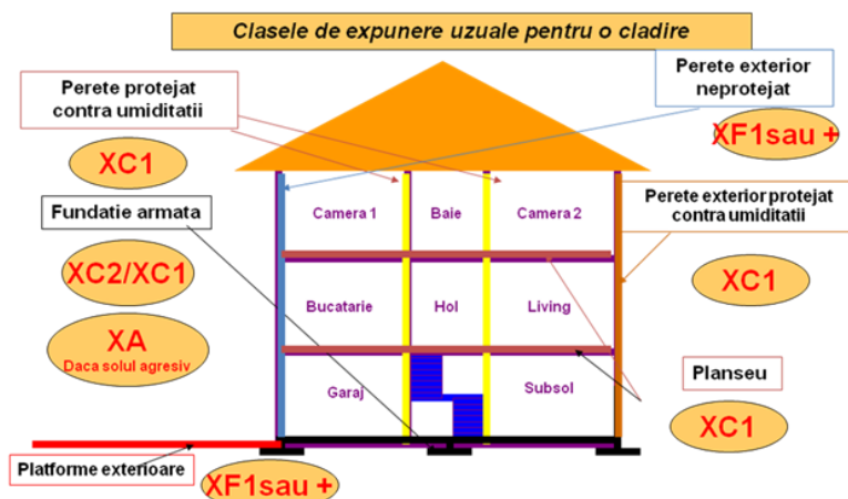
Рисунок V.5 - Примеры комбинации классов сред эксплуатации (гражданские здания)
