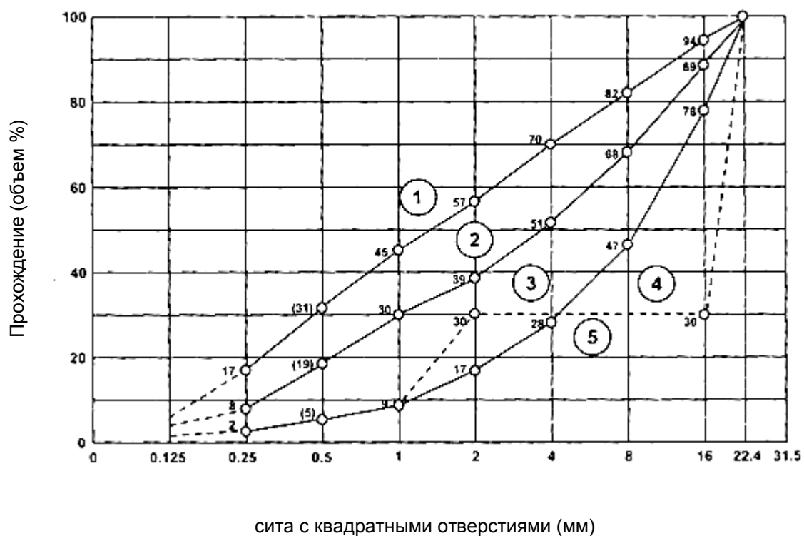
Рисунок J.2 - Гранулометрические области для максимального размера заполнителей 16 мм
