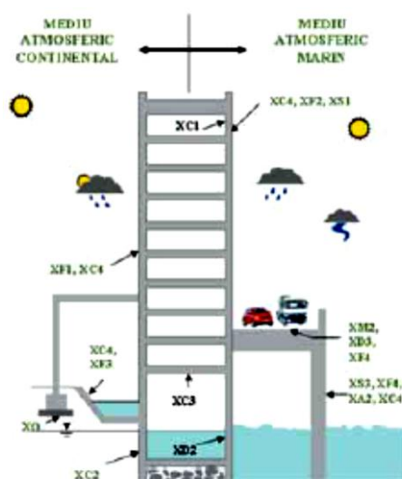
Figura V.4 - Exemple de combinații de clase de expunere pentru diferite tipuri de construcții și medii de expunere
