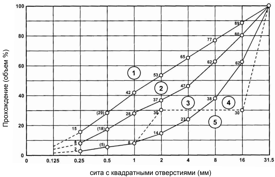
Рисунок J.3 - Гранулометрические области для максимального размера заполнителей 22 мм
