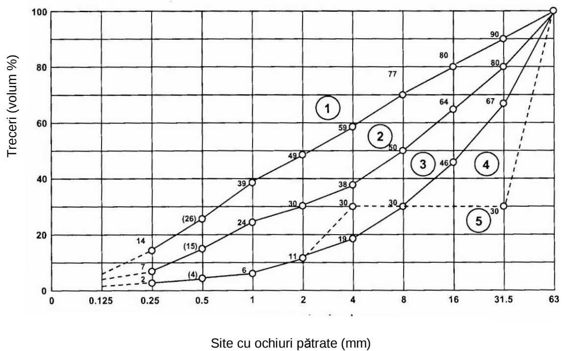
Figura J.4 - Zone de granulozitate pentru dimensiunea maximă a agregatelor de 32 mm
