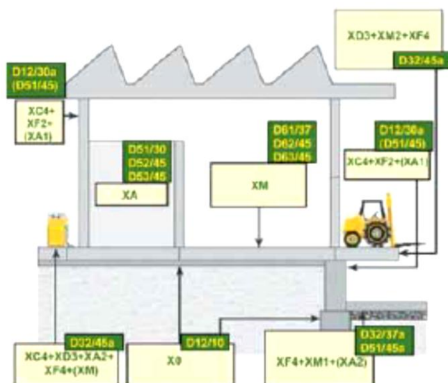
Figura V.3 - Exemple de clase de durabilitate / combinații clase de expunere (construcții industriale)
