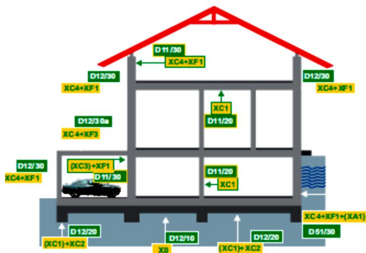
Рисунок V.1 – Примеры классов долговечности/комбинации классов сред эксплуатации (гражданские здания)
