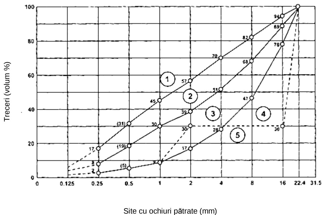
Figura J.2 - Zone de granulozitate pentru dimensiunea maximă a agregatelor de 16 mm
