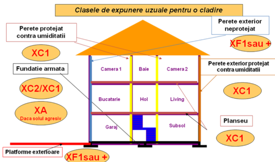
Figura V.5 - Exemplu de combinații de clase de expunere (construcții civile)
