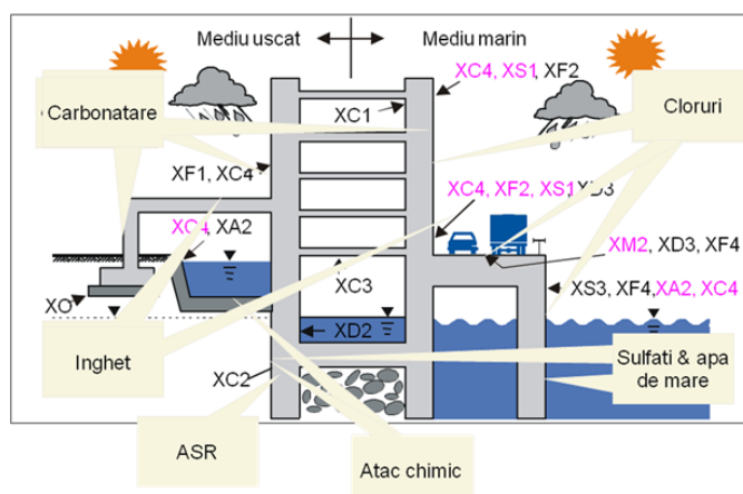
Figura V.6 - Exemple de combinații de clase de expunere pentru diferite tipuri de construcții și medii de expunere
