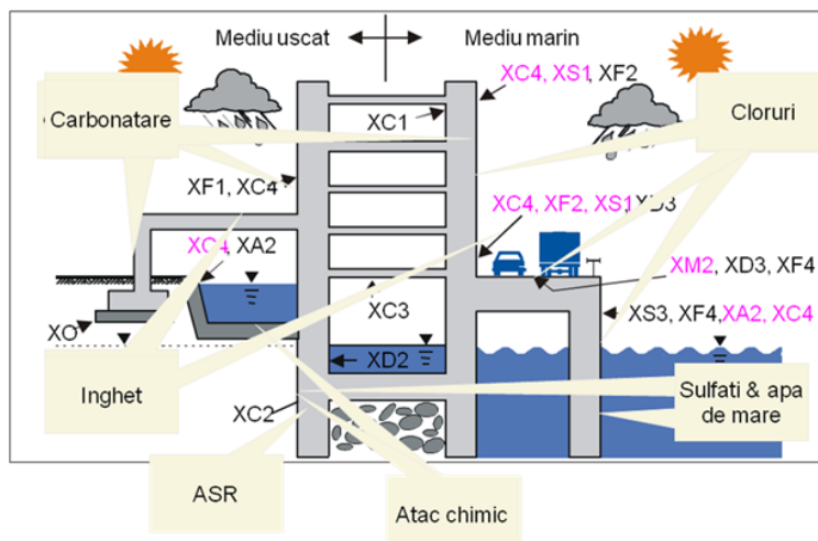
Рисунок V.6 - Примеры комбинаций классов сред эксплуатации для различных типов зданий и сооружений и сред эксплуатации
