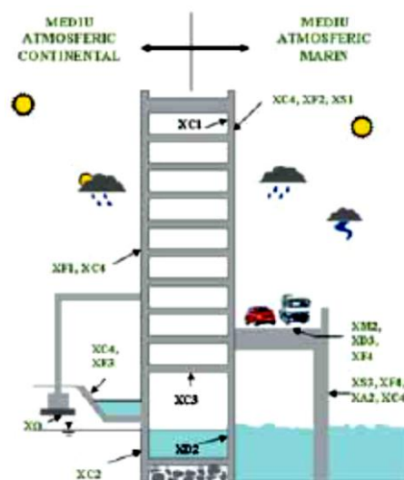
Рисунок V.4 – Примеры комбинаций классов сред эксплуатации для различных типов зданий и сооружений и сред эксплуатации
